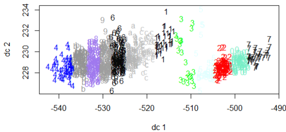
Figura 33 (a) Gráfico de cada experimento para agrupar os Clusters de acordo com suas similaridades no algoritmo K-Means para 13 Clusters . Experimento #1: Média com filtro.
